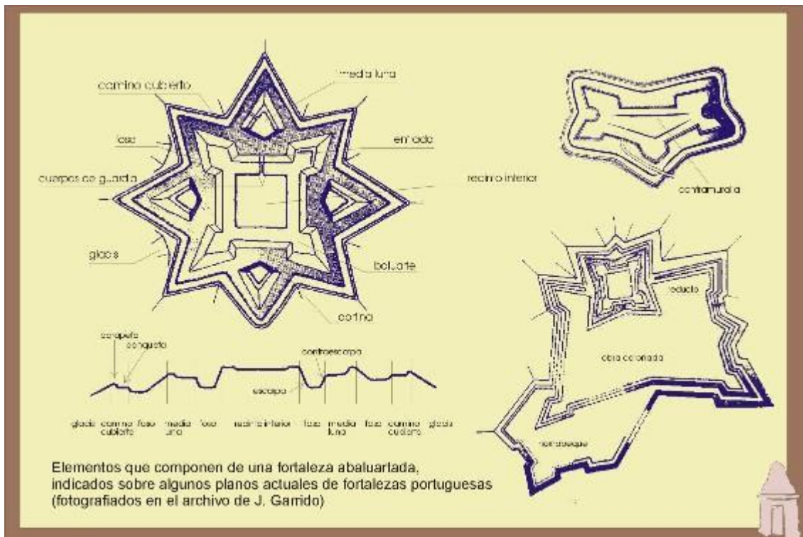
FIG 9. Elementos que componen una fortaleza abaluartada.
