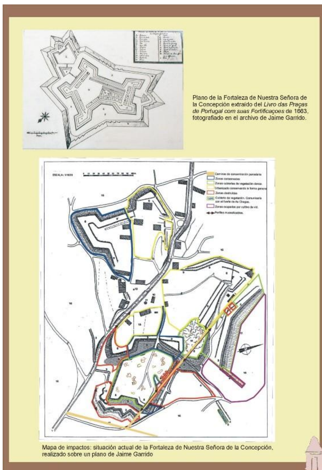
FIG 17. Sistema Goián-Medos-Vilanova de Cerveira: análisis de la planimetría histórica de la Fortaleza de Nossa Senhora da Conceição y estado actual de la misma.
