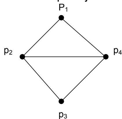
Figura 4. Un grafo con cuatro puntos y cinco aristas
